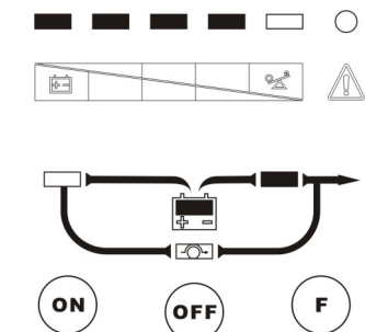
Рисунок 4-2 Режим работы от батарей
