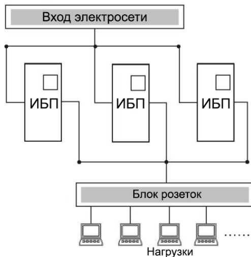
Схема параллельного подключения ИБП
