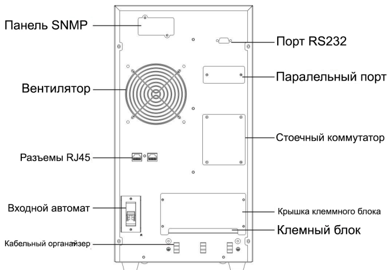
Задняя панель ИБП Pro 6H3
