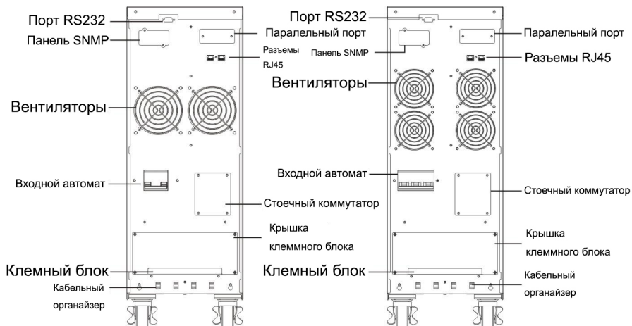
Задняя панель Pro 10S3
