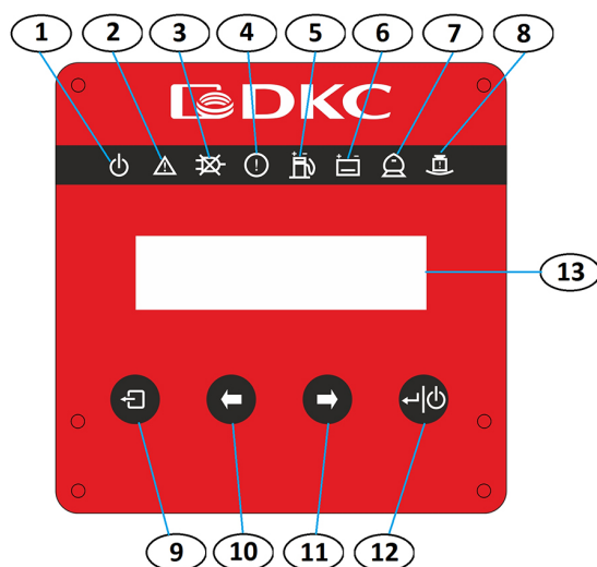
Рисунок 2 – Передняя панель ИБП
