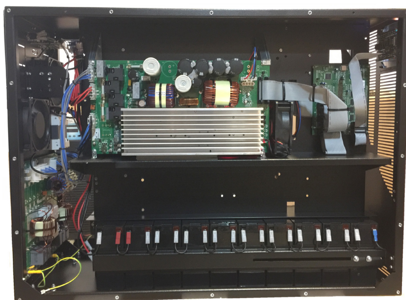
Рисунок 5 – Расположение батарей 7/9 Ач Trio TT
