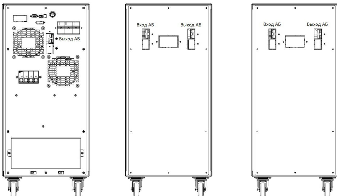
Рисунок 7 – Подключение внешних батарейных блоков к ИБП серии Trio TT
