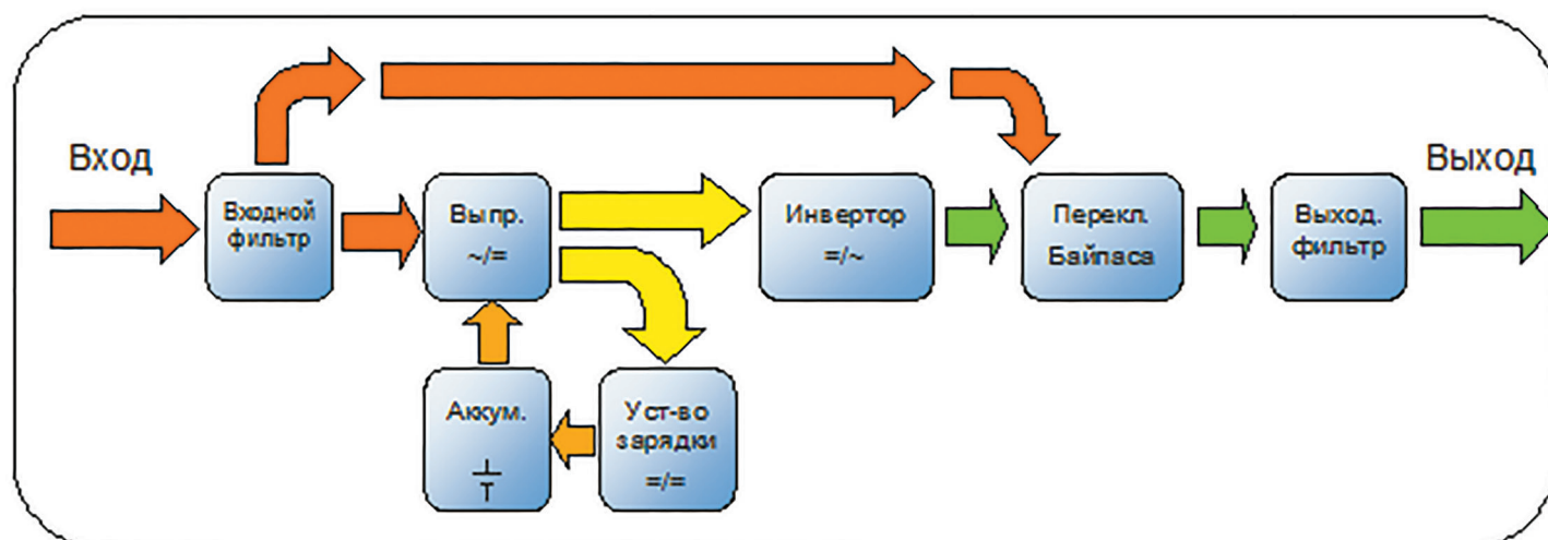
Рисунок 1 – Блок-схема
