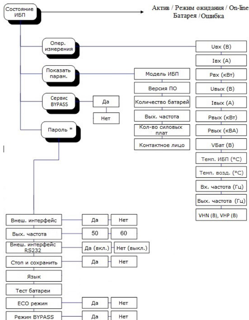
Рисунок 3 – Блок-схема ПО ИБП
