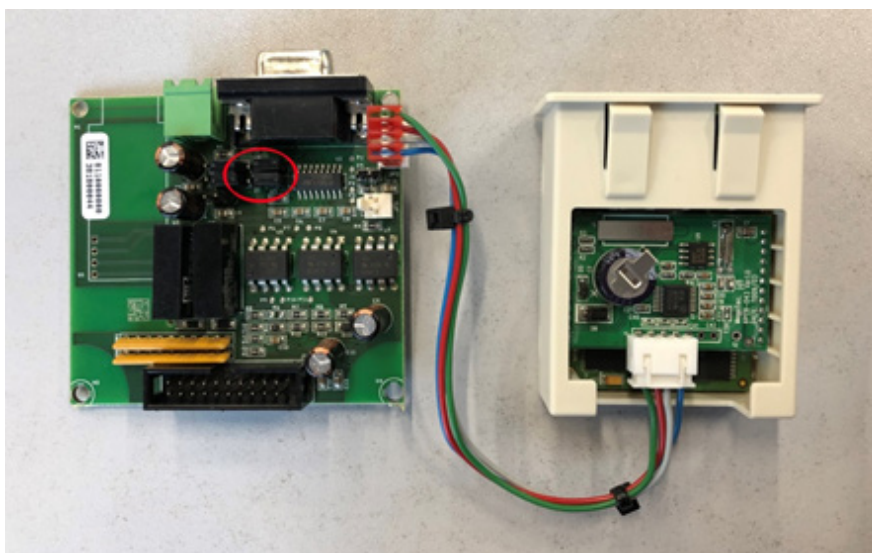
Рисунок 9 – Подключение платы SNMP
