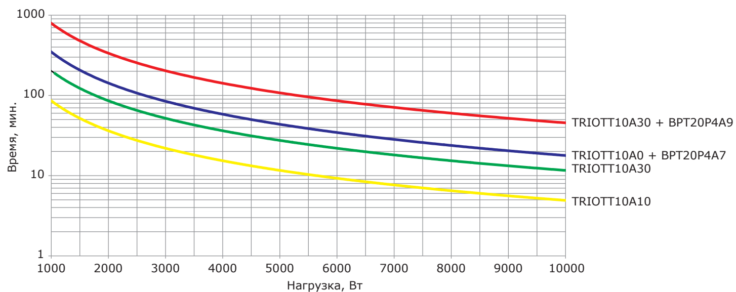
Рисунок 5 – Разрядные характеристики модели TRIOTT10
