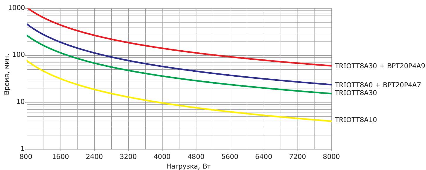
Рисунок 4 – Разрядные характеристики модели TRIOTT8
