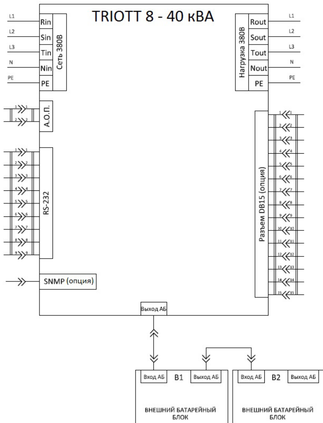
Рисунок 4 – Схема подключения ИБП серии Trio TT
