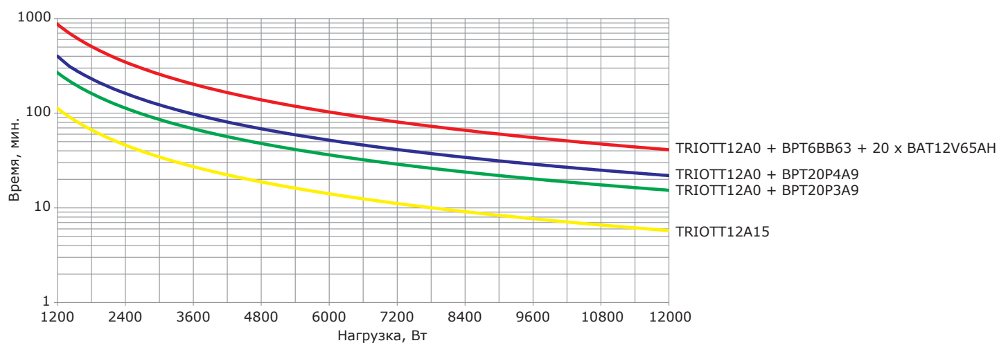
Рисунок 6 – Разрядные характеристики модели TRIOTT12
