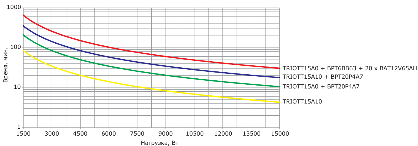
Рисунок 7 – Разрядные характеристики модели TRIOTT15
