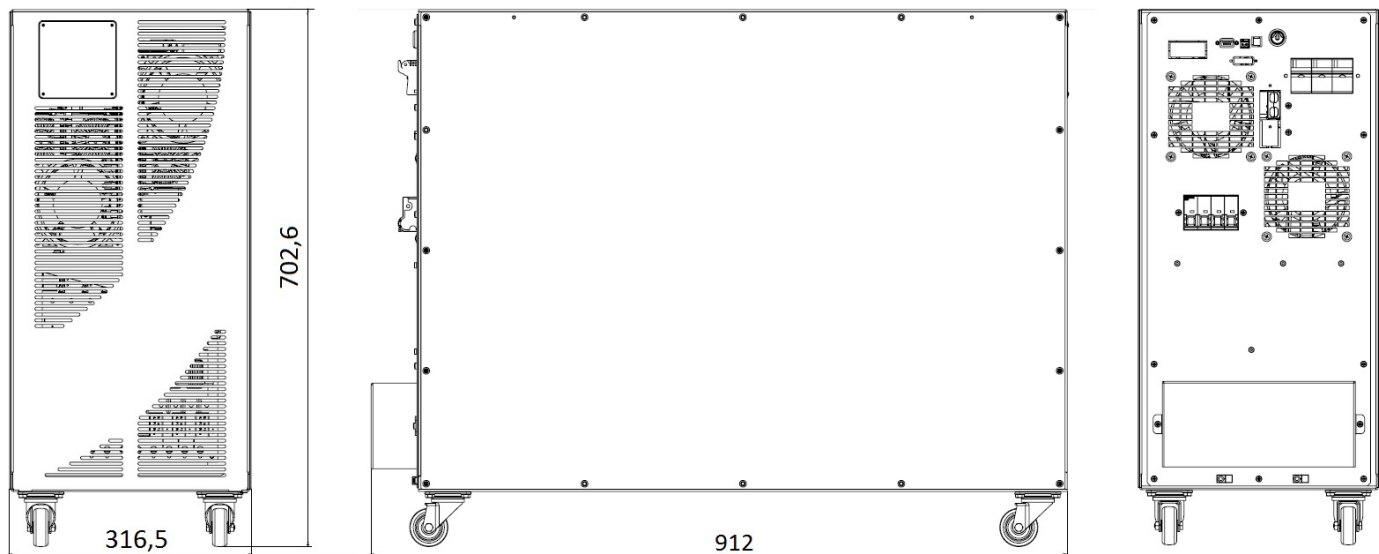
Рисунок 1 – Внешний вид ИБП серии Trio TT
