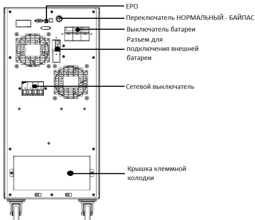
Рисунок 3 – ИБП серии Trio TT, вид сзади
