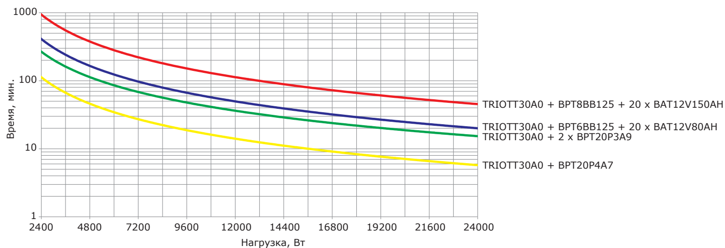
Рисунок 9 – Разрядные характеристики модели TRIOTT30
