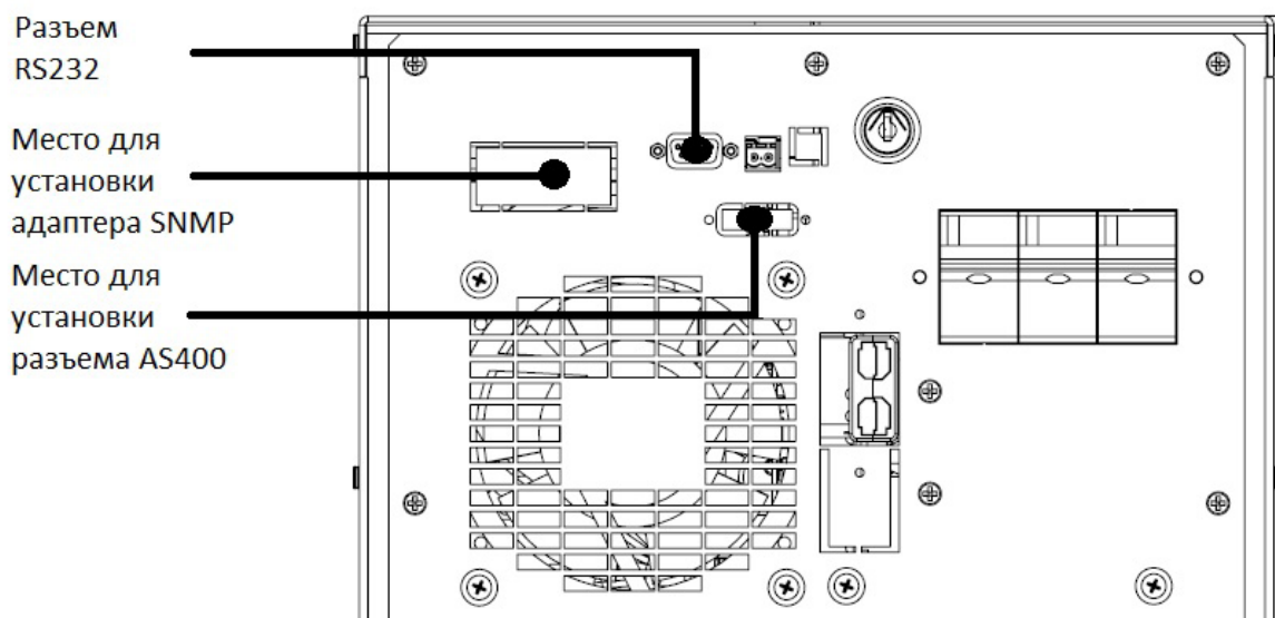
Рисунок 8 – Интерфейсы Trio TT
