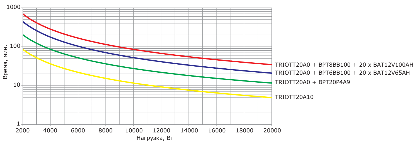
Рисунок 8 – Разрядные характеристики модели TRIOTT20
