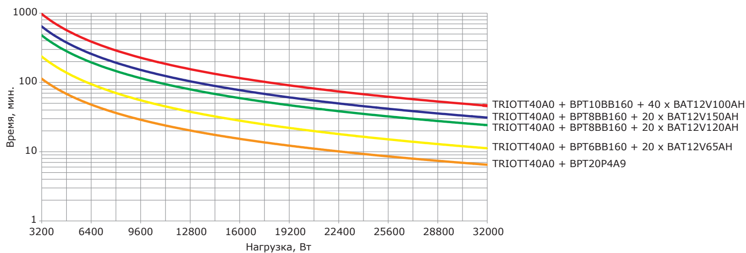
Рисунок 10 – Разрядные характеристики модели TRIOTT40
