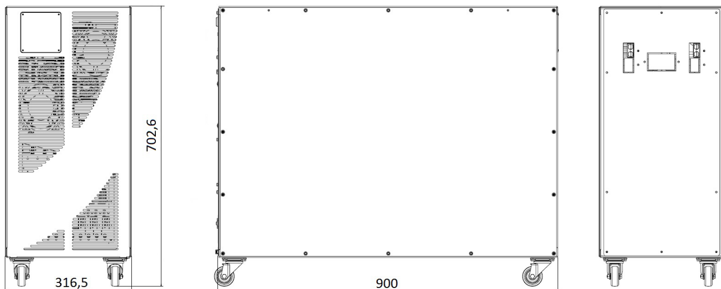
Рисунок 2 – Размеры внешнего батарейного шкафа серии Trio TT
