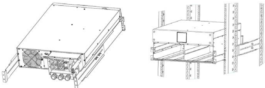
Рисунок 3-12. Установка выдвижных рельсов
