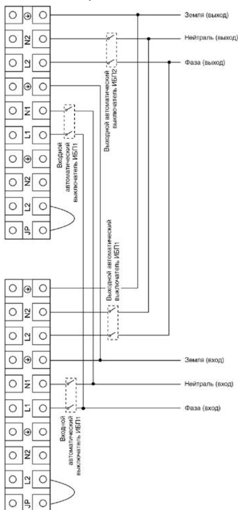
Рисунок 4-5.a. Схема параллельного подключения для 6К/10К
