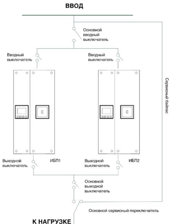
Рисунок 4-5.b. Схема параллельной установки
