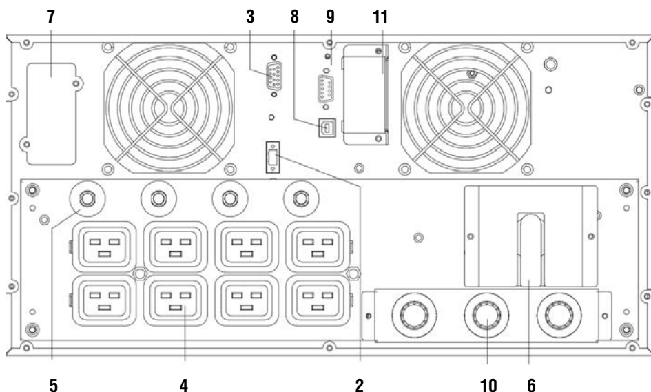
Рисунок 3-6. Задняя панель модели Online RT 10K
