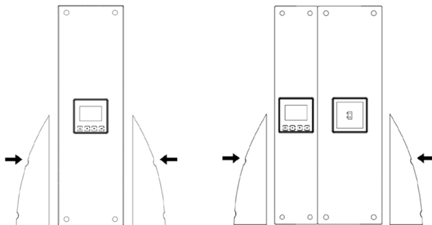
Рисунок 3-17. Вертикальная установка
