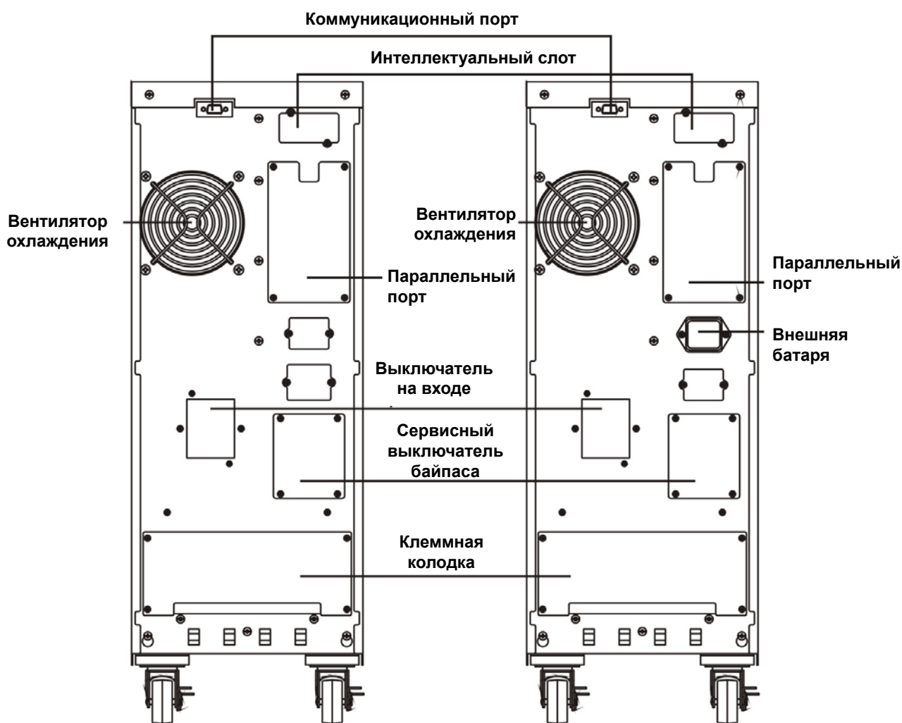
Вид сзади модели 6000HXL
