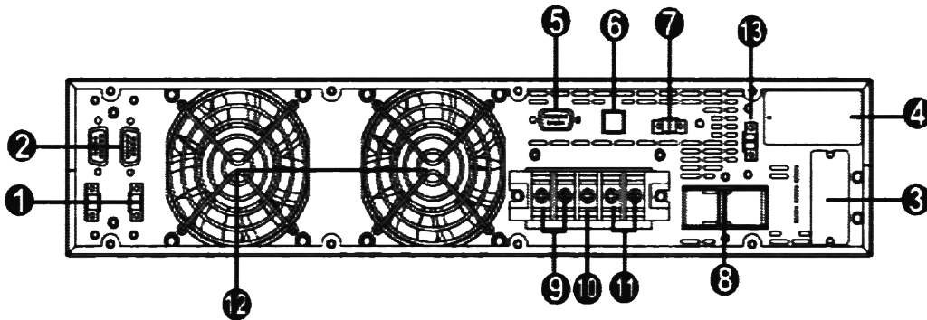
Рис.1 Задняя панель
