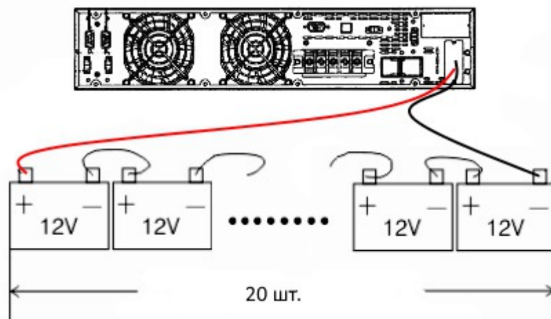
Схема подключения комплекта внешних АКБ.
