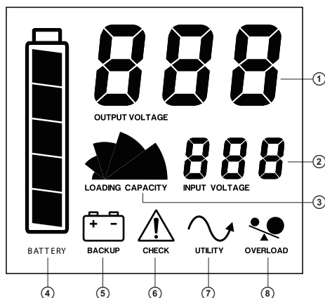
Рис. 1. LCD-дисплей ИБП
