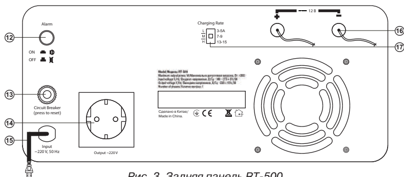
Рис. 3. Задняя панель RT-500
