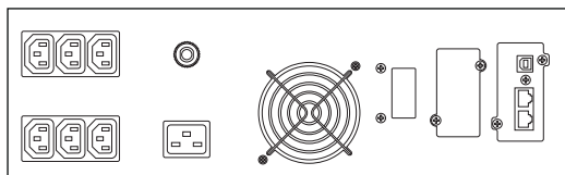
Задняя панель ИБП в стойку ЮНИОР ПРО РТ 2000 и 3000 ВА 3U
