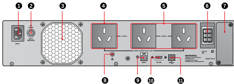
Задняя панель: UPS102R2RT0B0B2
