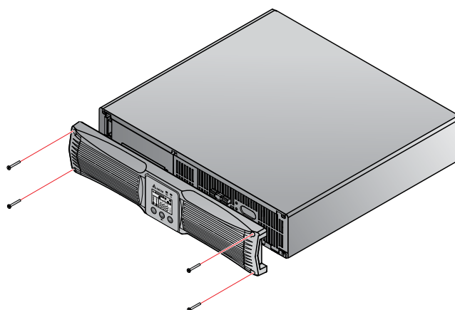
Рис. 3-5. Снимите пластмассовую переднюю панель
